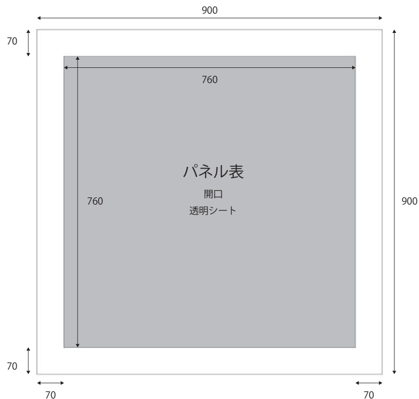
正面パネル
